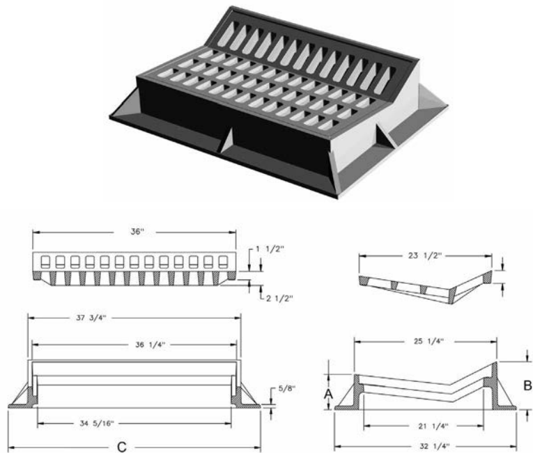
V-4510 — V-4516 Gutter Inlet
